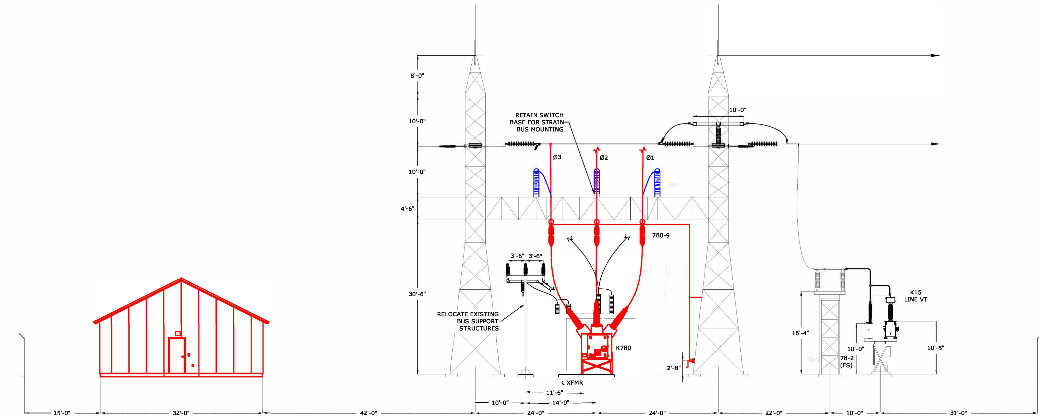
ELEVATION B-B
