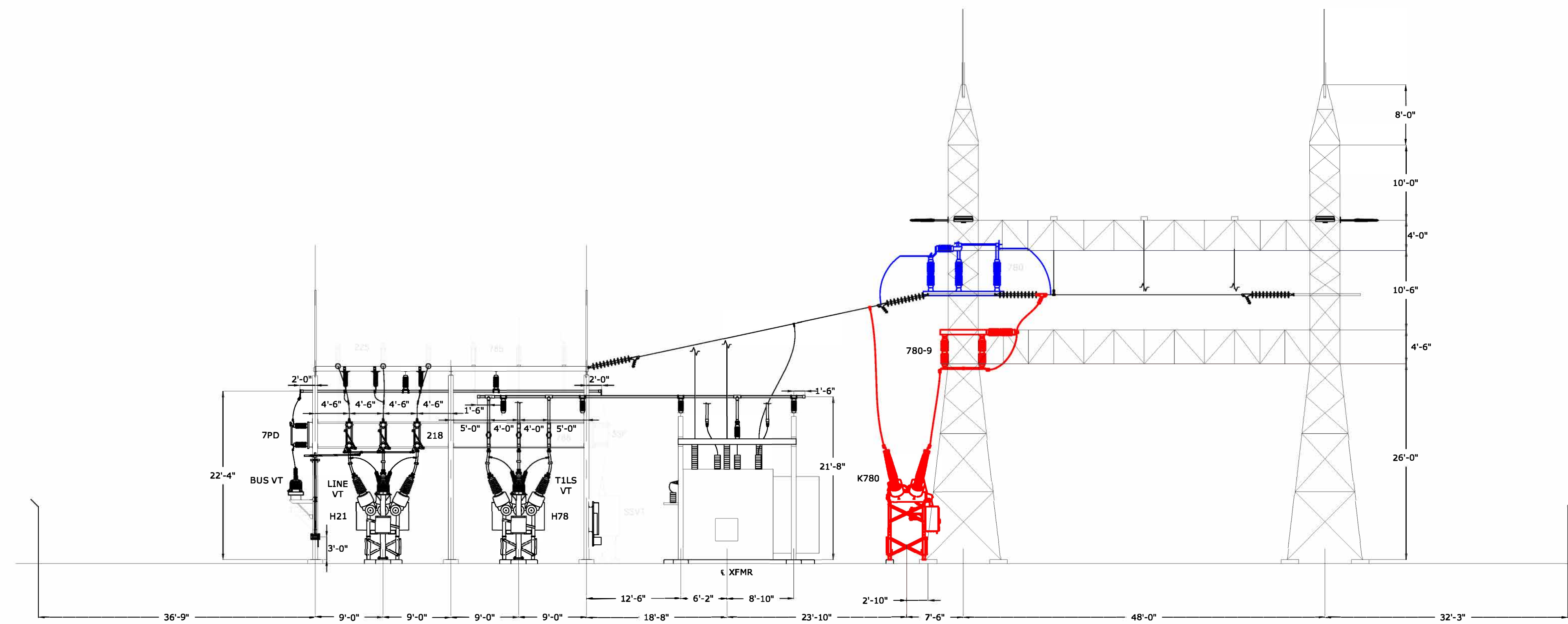
ELEVATION A-A
